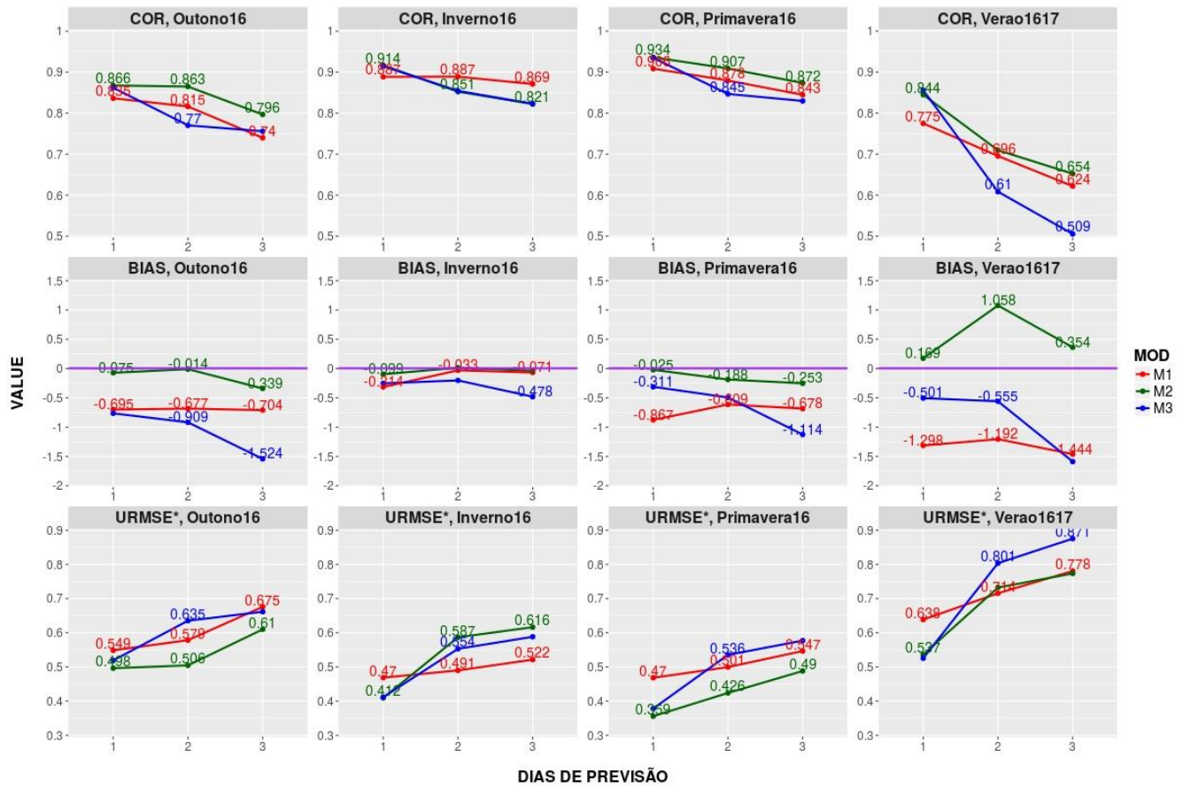
Figura C5. Idem à Figura C1 para a região La Plata
