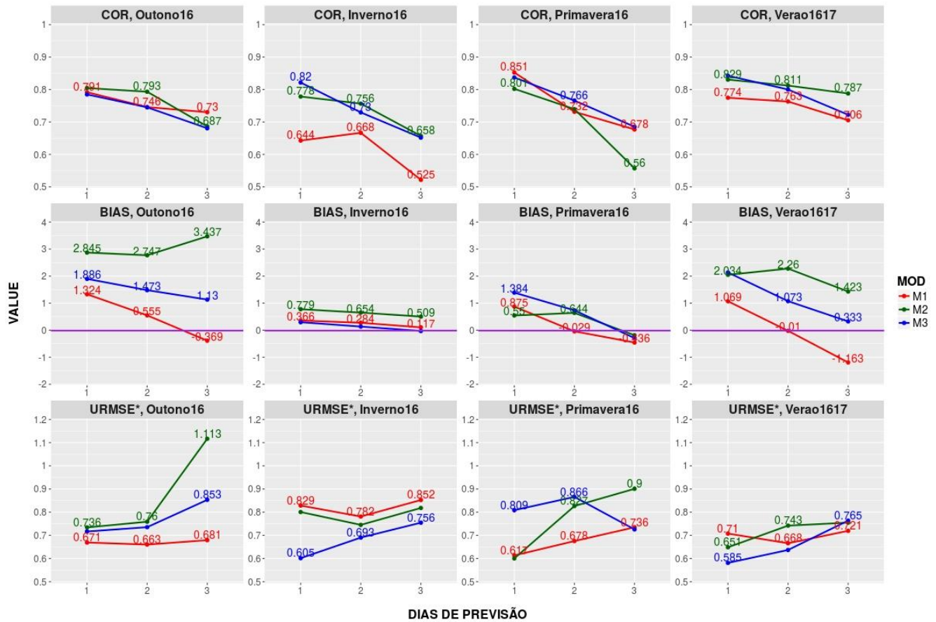
Figura C3. Idem à Figura C1 para a região Nordeste.
