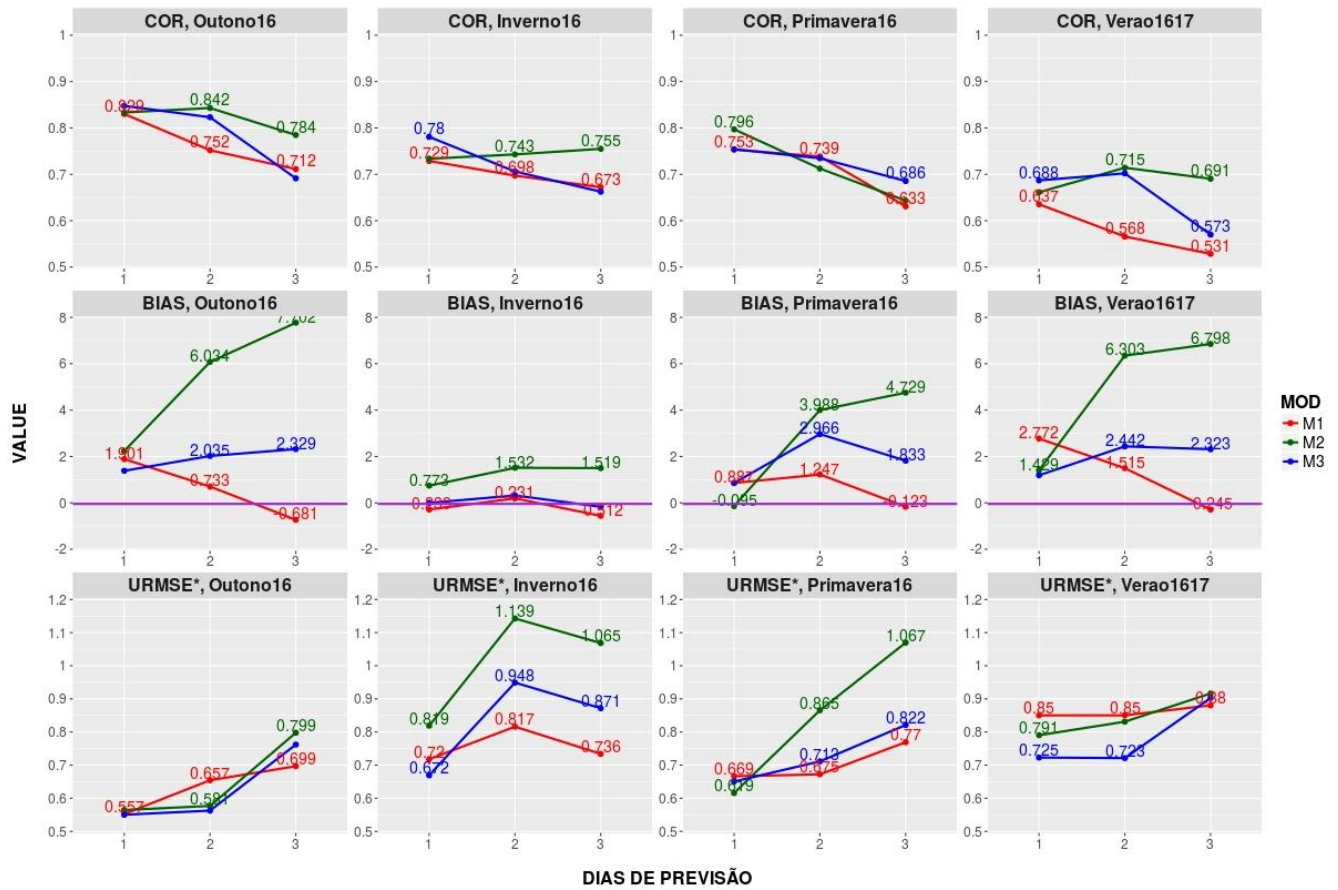
Figura C1. Correlação, Vies e RMSE* entre a precipitação prevista e observada para a região Amazônica.
