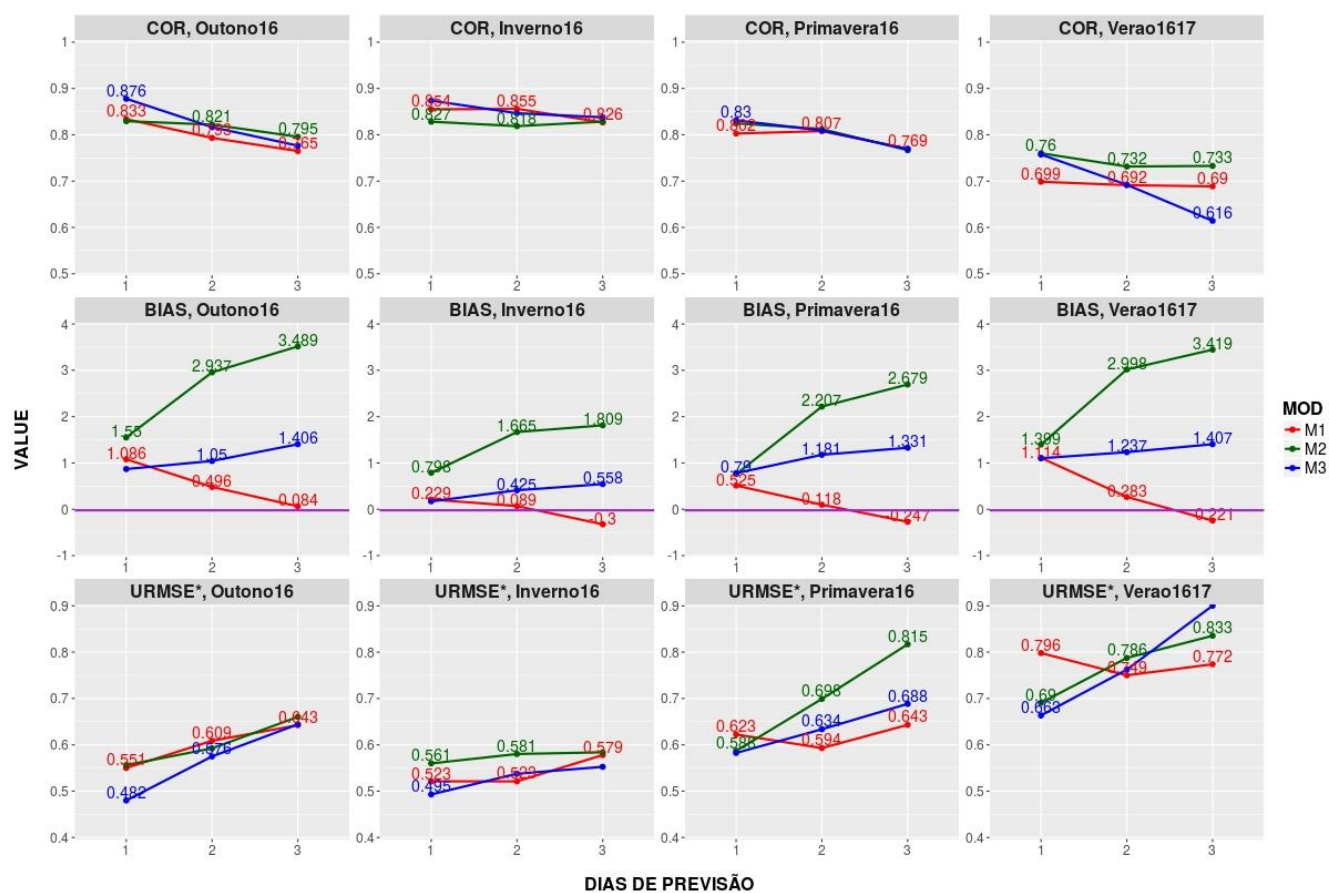
Figura C6. Idem à Figura C1 para a região América do Sul
