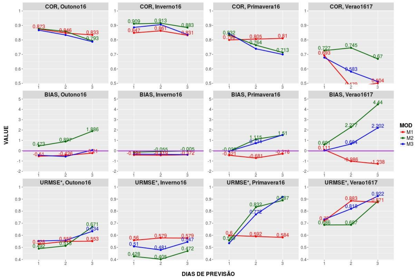
Figura C2. Idem à Figura C1 para a região Centro-Oeste.
