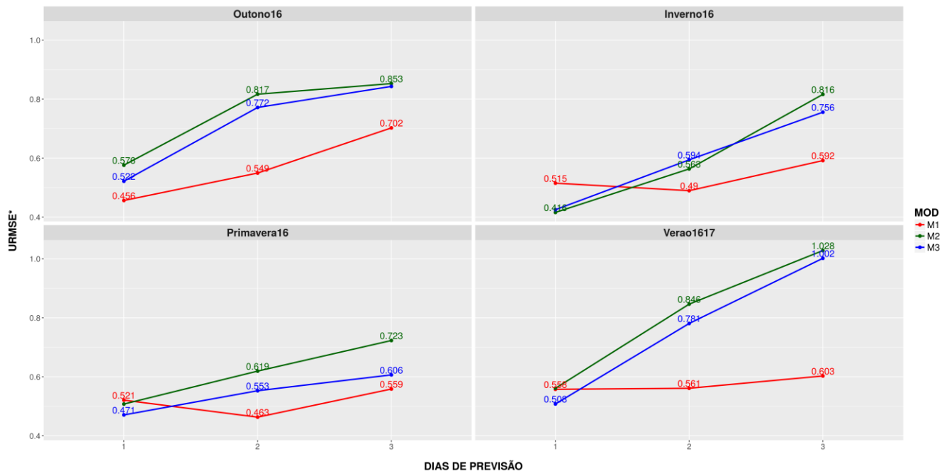
Figura C4. Idem à Figura C1 para a região Sudeste
